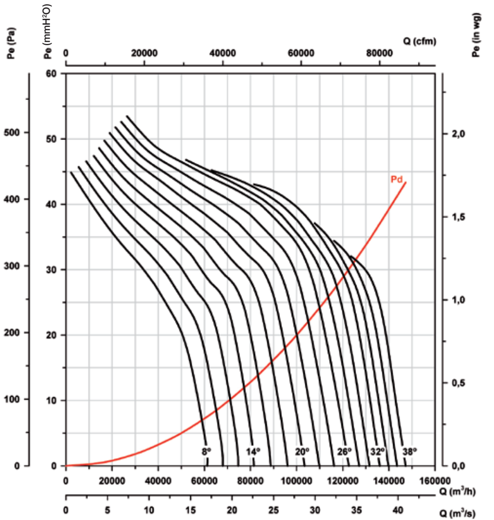
Potencia absorbida
