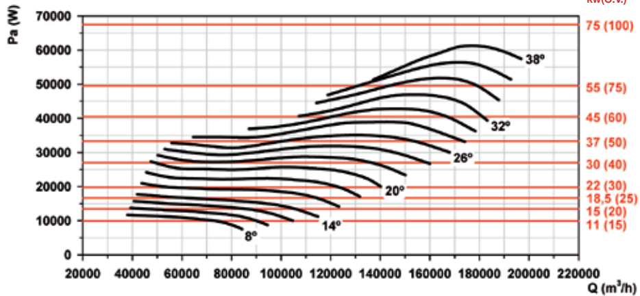
Potencia absorbida
